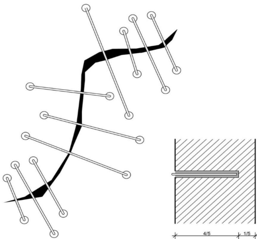
☒ Schématické usporiadání skob při stehování trhliny
